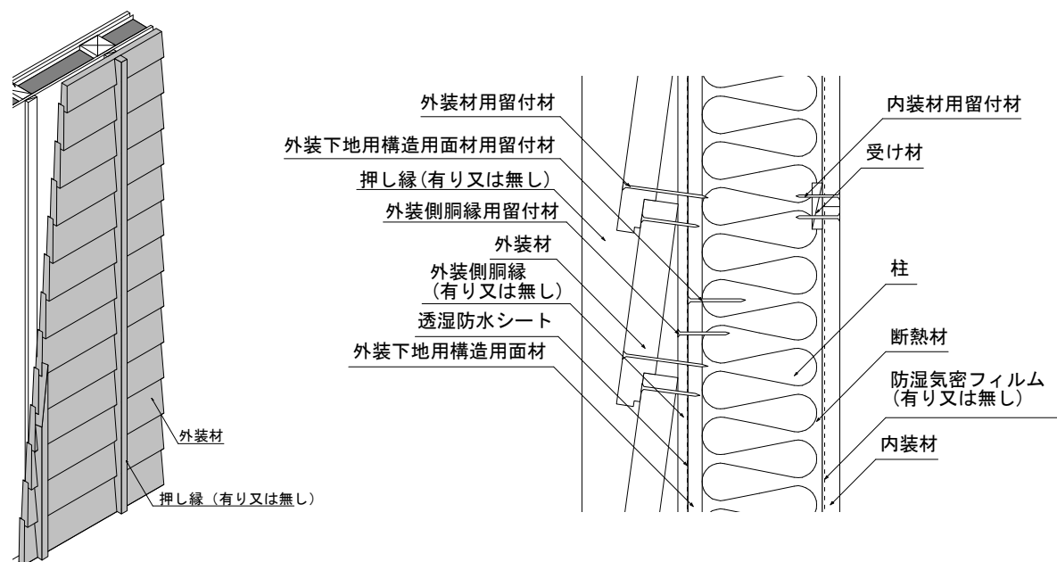
横張り (下見板張り)
