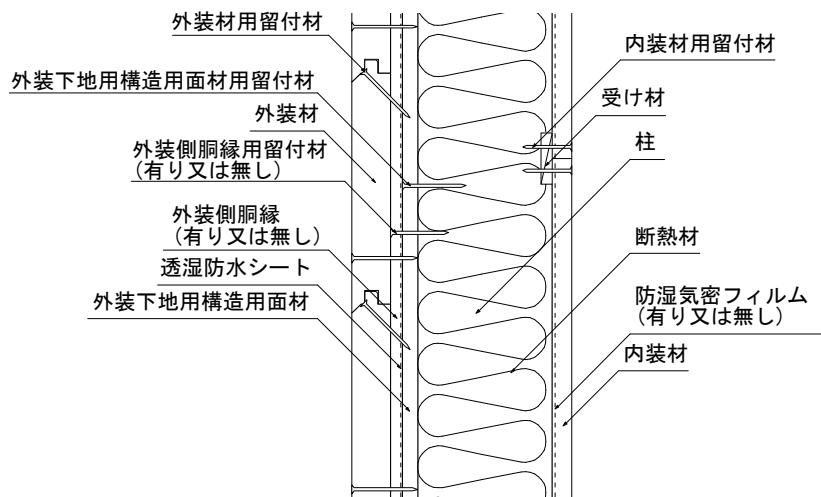
横張り（本実張り）鉛直断面図
