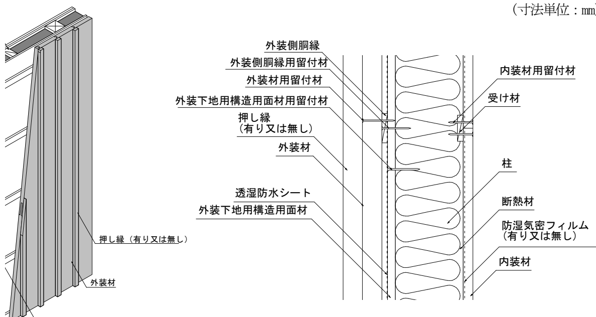
縦張り (本実張り)
